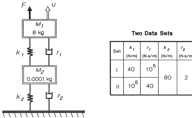
a. Structure and Parameters
