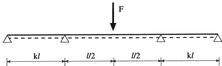
Fig. 1. Stüssi-Kollbrunner beam.
