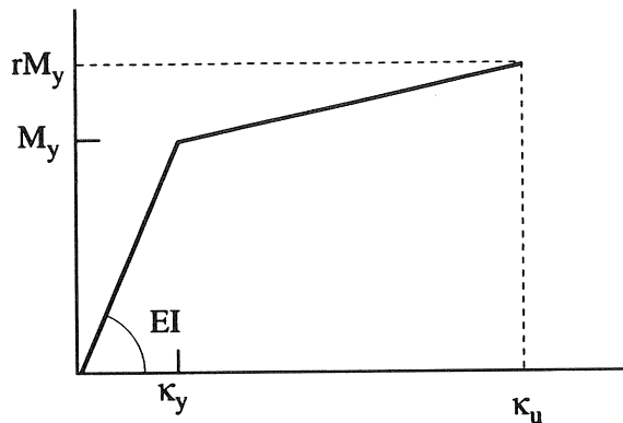
Fig. 5. M - \kappa -diagram.
