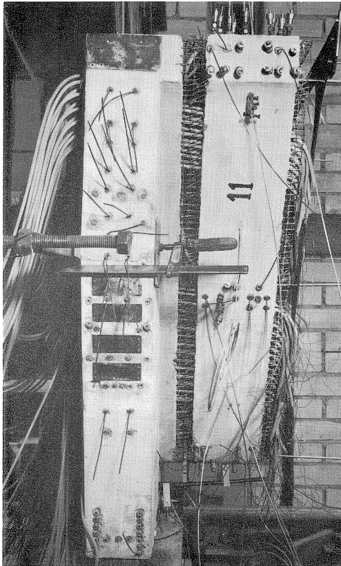
Fig. 14. Overzicht van de wijze, waarop de spelingen voor de kabels in lengterichting ter plaatse van de voegen werden verkregen. Tevens zijn enkele verankeringen van de kabels in dwarsrichting te zien.
