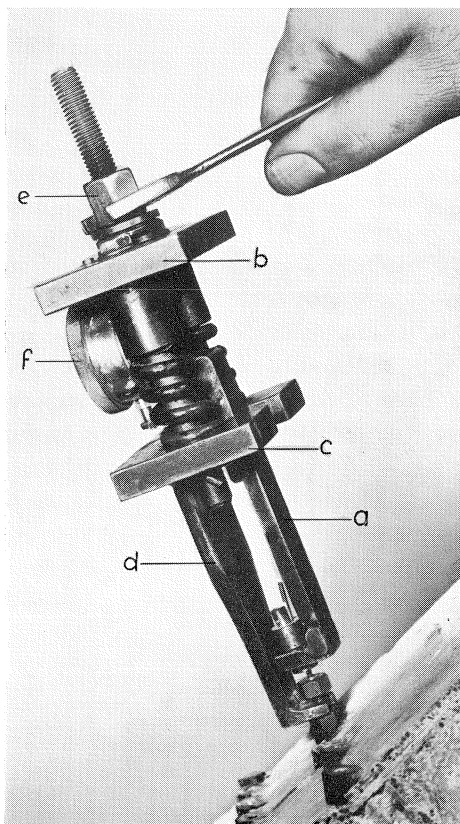
Fig. 16. Het spanapparaat voor de kabels in dwarsrichting.
