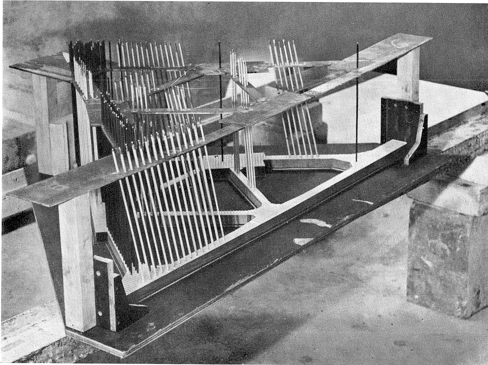
Fig. 7. Overzicht van de wijze, waarop de spelingen voor de kabels in lengterichting werden verkregen en gefixeerd.
