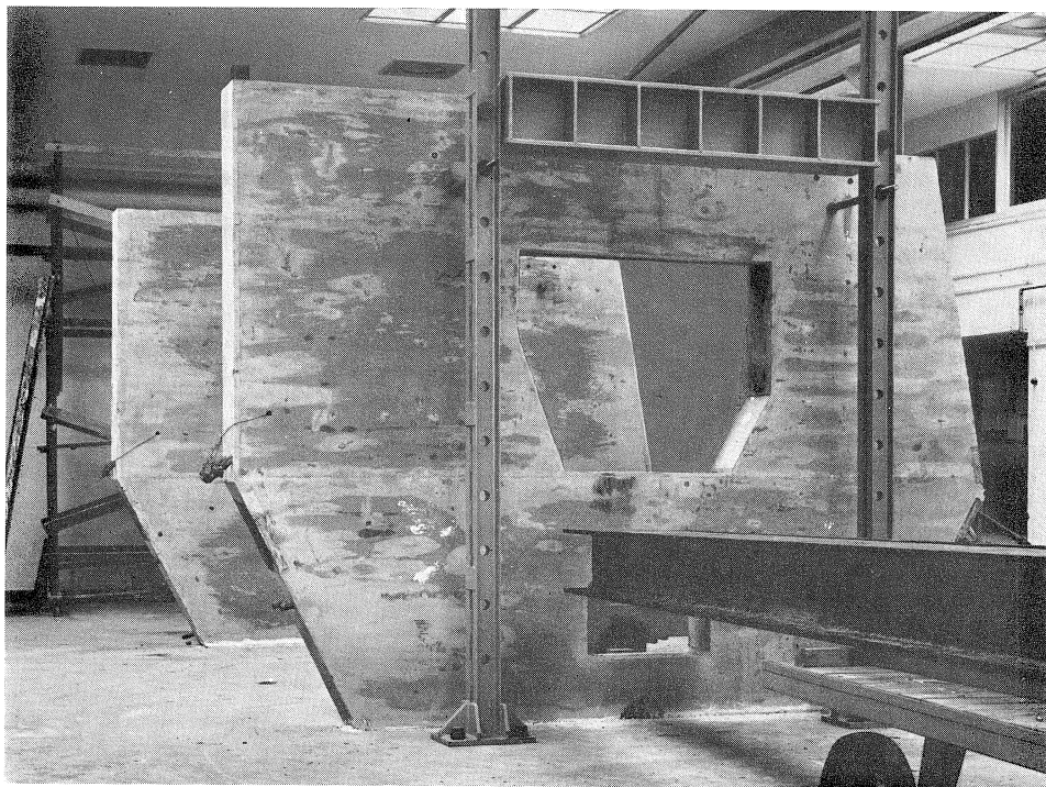
Fig. 18. De bij het model toegepaste pijlerconstructie.
